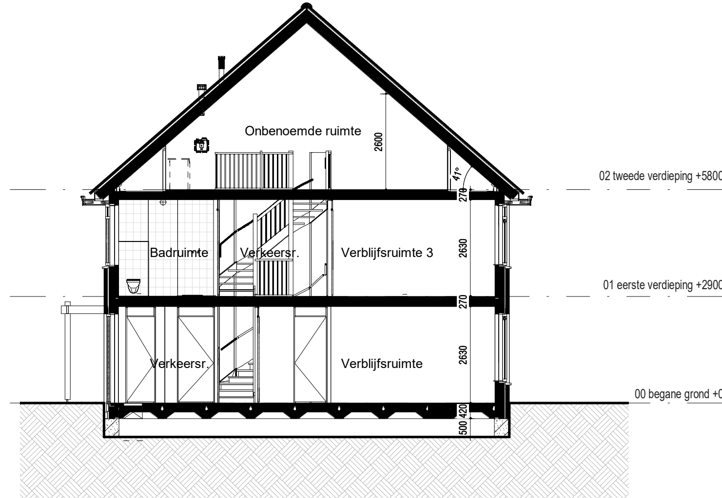
Doorsnede (1:100)
