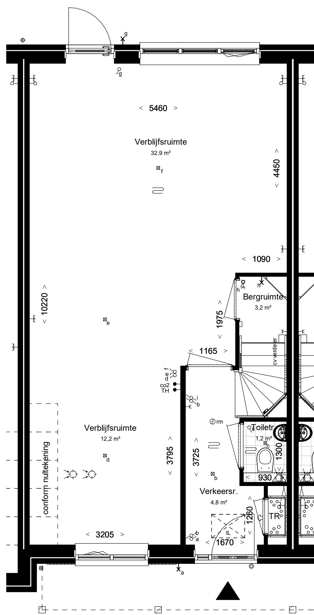
Begane grond, PEIL=0 Woningtype: 3.0_sp Beukmaat: 5700
