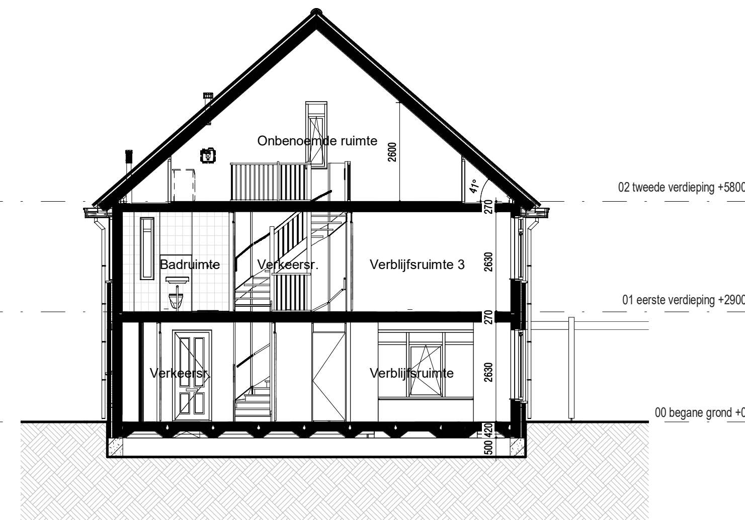
Doorsnede (1:100)
