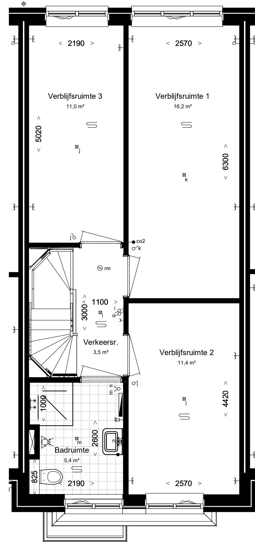
Eerste verdieping, 2900+P
