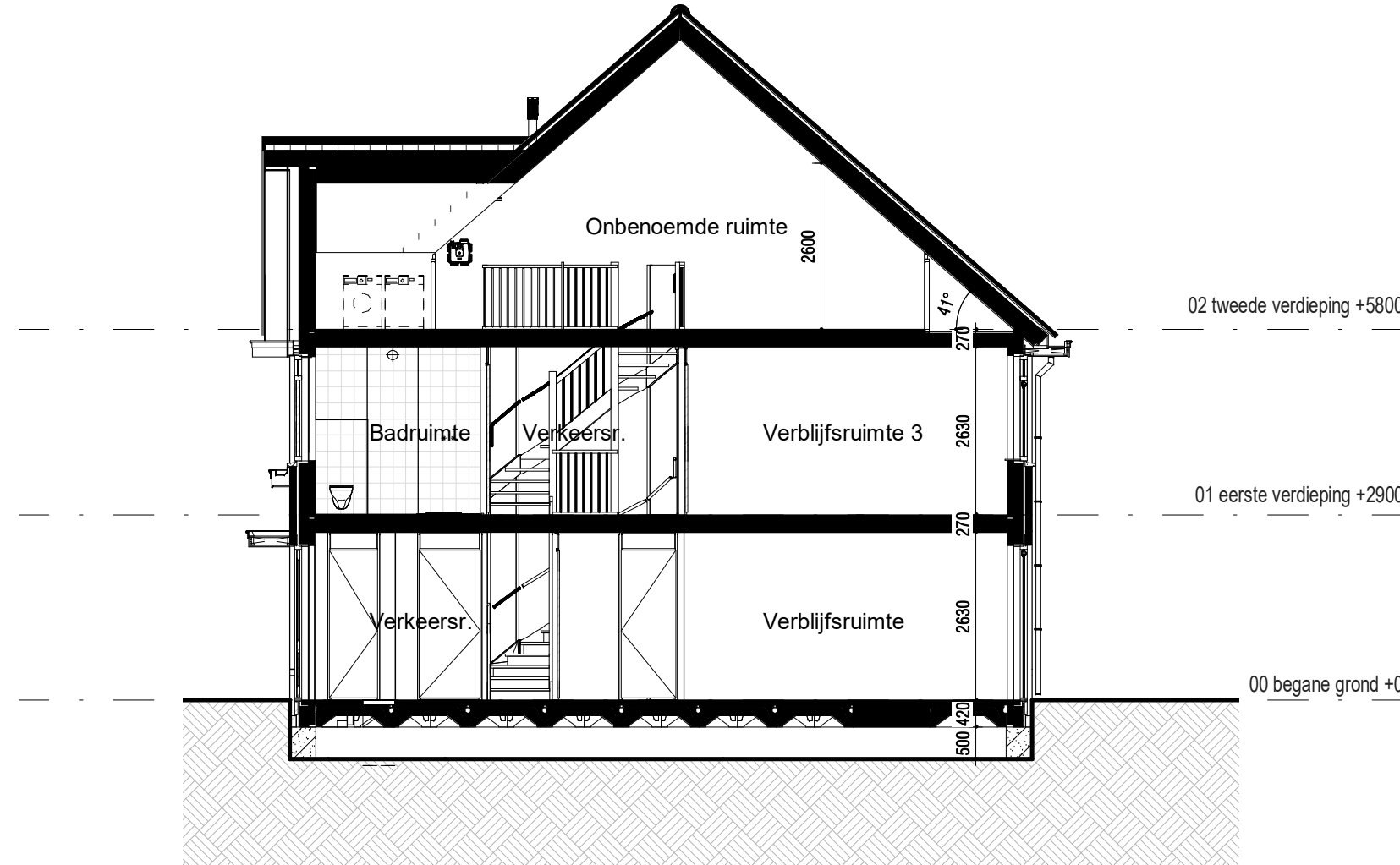
Doorsnede (1:100)
