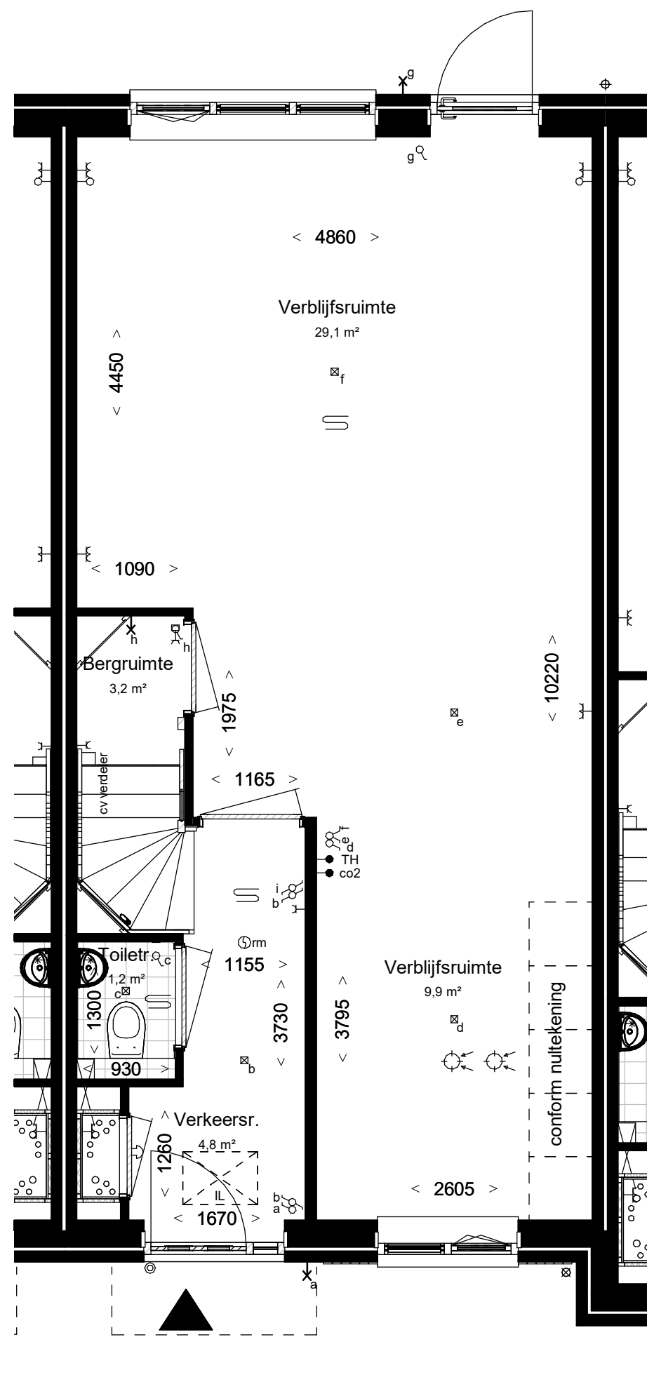
Begane grond, PEIL=0 Woningtype: 1.0 Beukmaat: 5100
