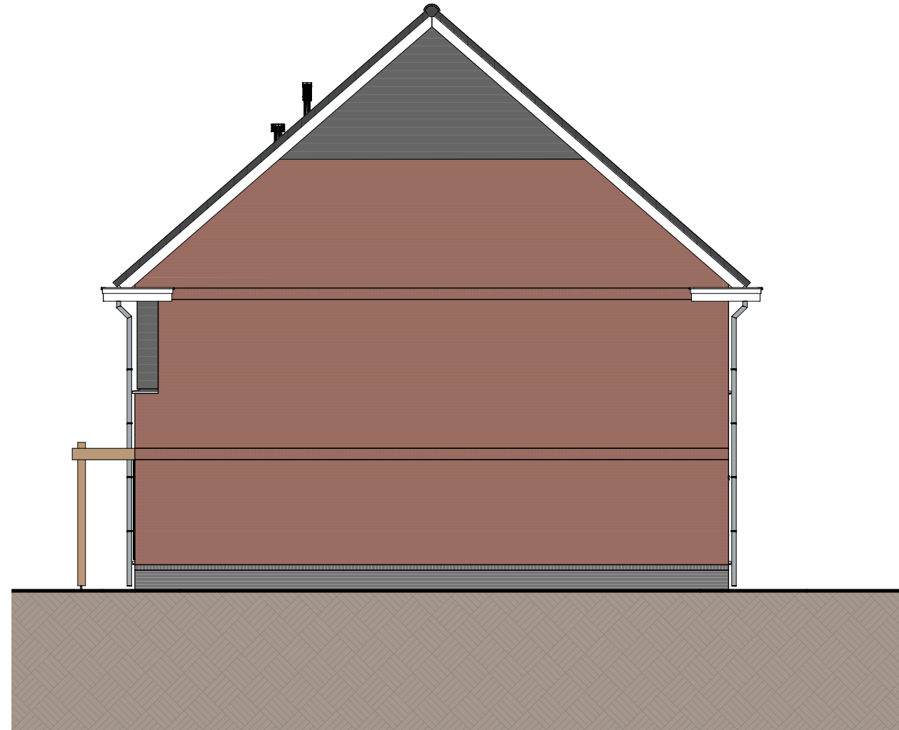
Rechter zijaanzicht (1:100)
