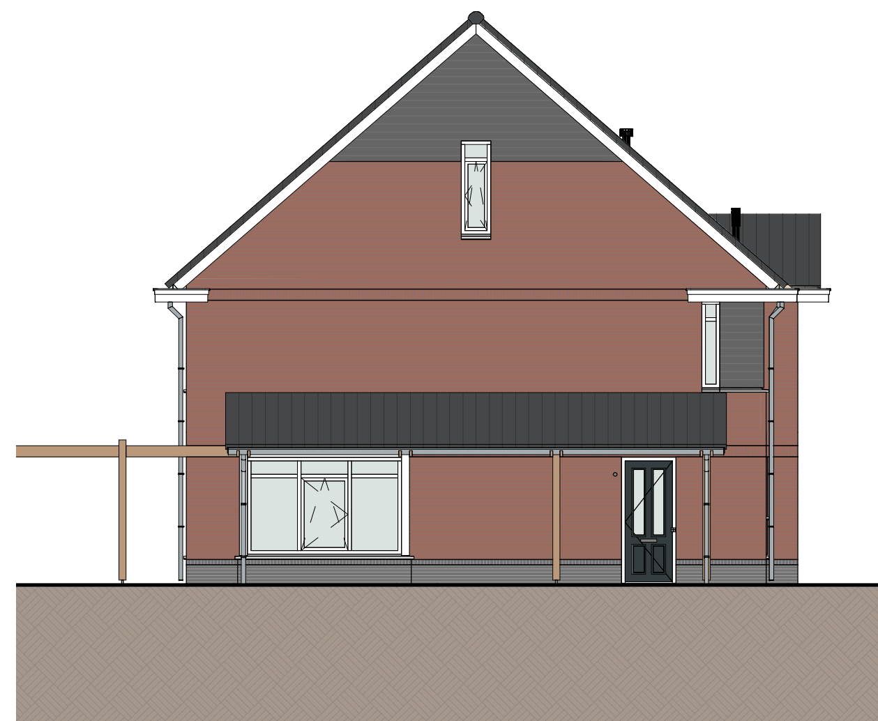
Linker zij aanzicht (1:100)
