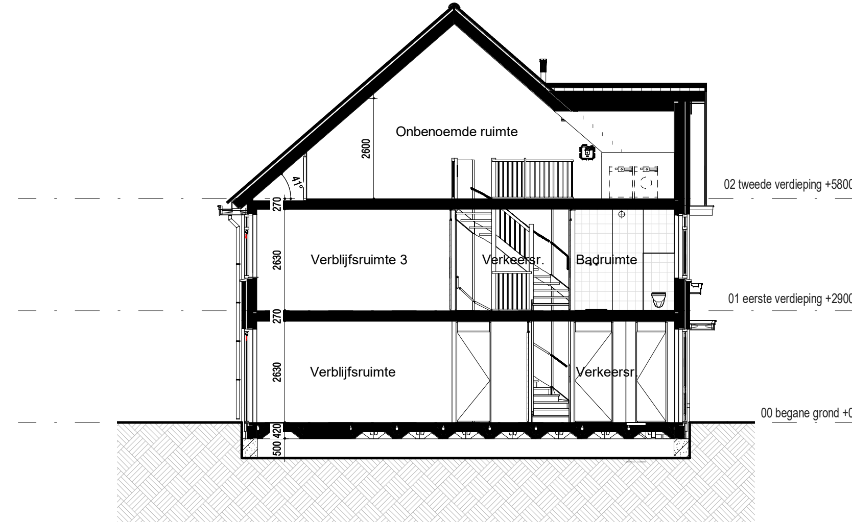
Doorsnede (1:100)
