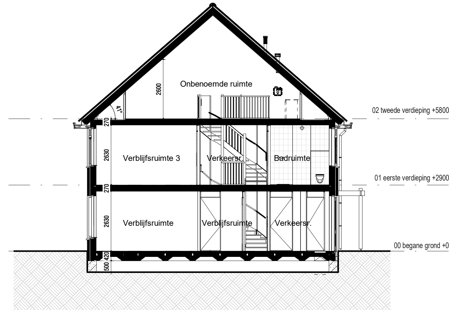
Doorsnede (1:100)
