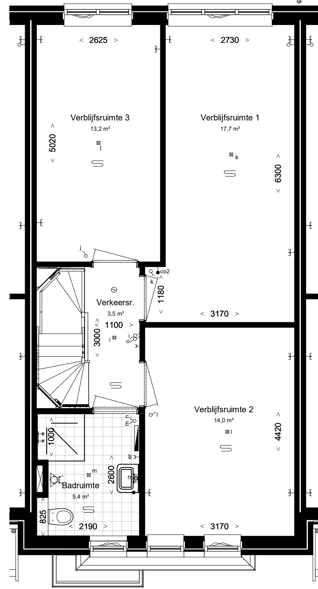
Eerste verdieping, 2900+P
