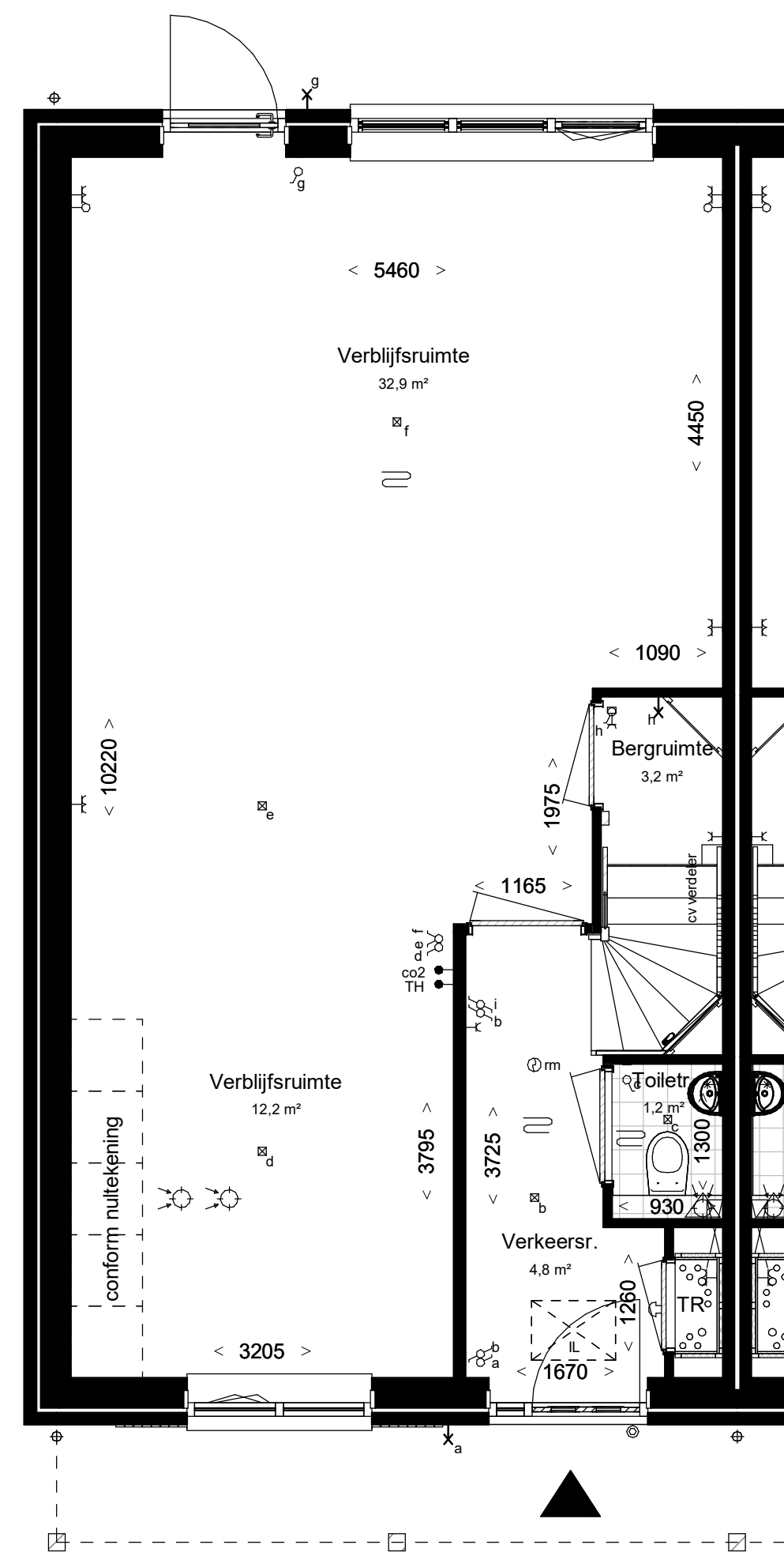
Begane grond, PEIL=0 Woningtype: 3.8_sp Beukmaat: 5700
