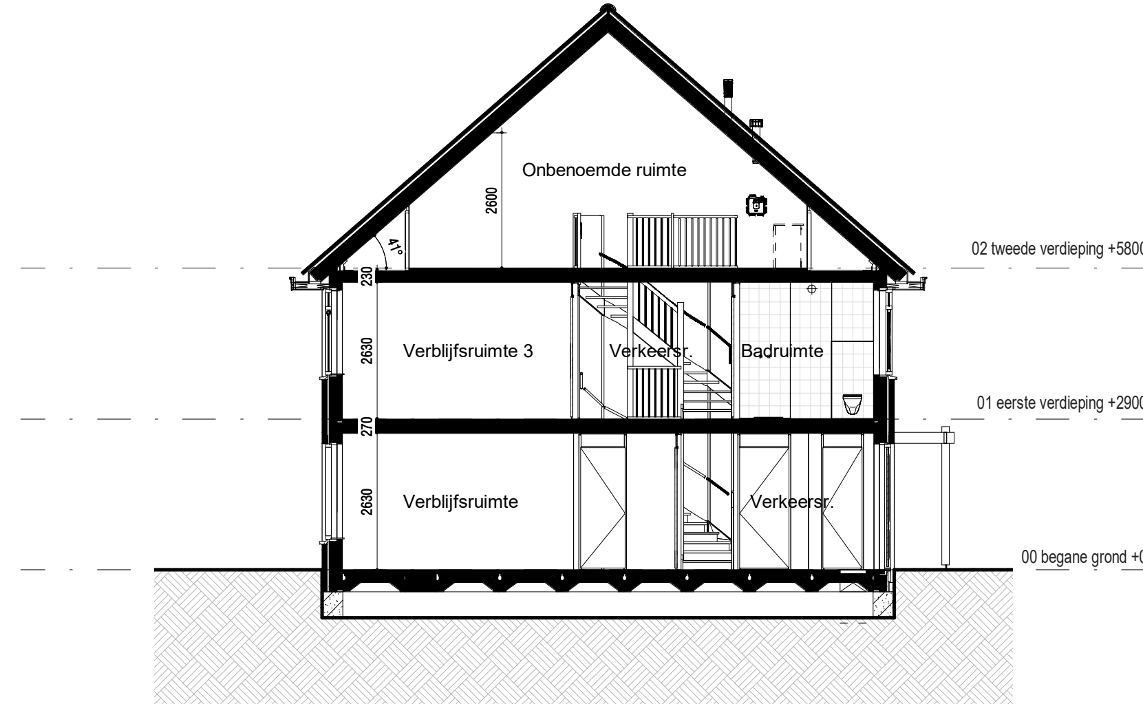
Doorsnede (1:100)
